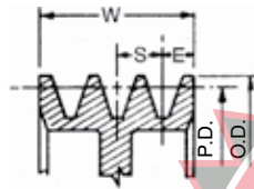
Groove Dimensions
