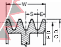
Groove Dimensions
